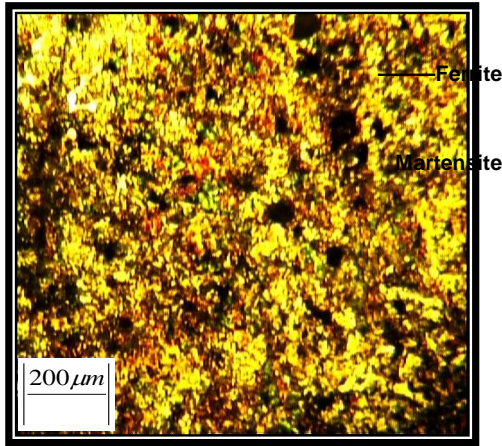
الشكل (٢٠) معدن اللحام (WM) لعينه سمك (2mm) ولزمن (8sec) وغاز CO 2 .
