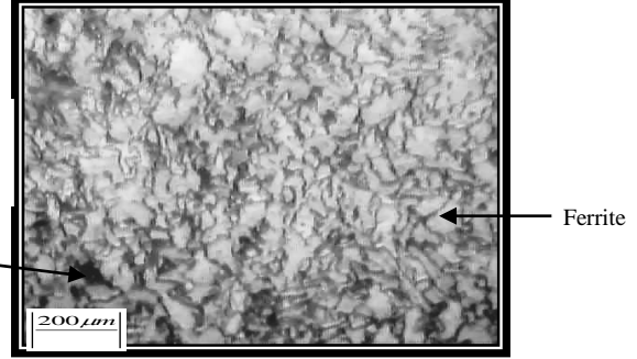
الشكل (١٧) صورة التركيب المجهرى الدقيق للمعدن الأساس DIN15Mo3
