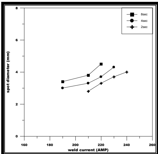
الشكل (١٠) تأثير التيار في قطر نقطة اللحام لسمك 2mm مع استخدام غاز Ar ولازمان مختلفه
