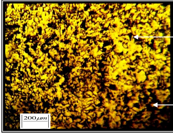
الشكل (١٩) معدن اللحام (WM) لعينه سمك (2mm) لزمن (4sec) وغاز CO 2
