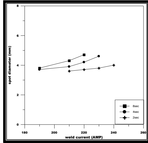
الشكل (٧) تأثير التيار في قطر نقطة اللحام لسمك 2mm مع استخدام غاز CO 2 ولازمان مختلفه
