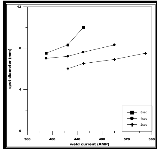
الشكل (١٢) تأثير التيار في قطر نقطة اللحام لسمك 4mm مع أستخدام غاز Ar ولازمن مختلفه
