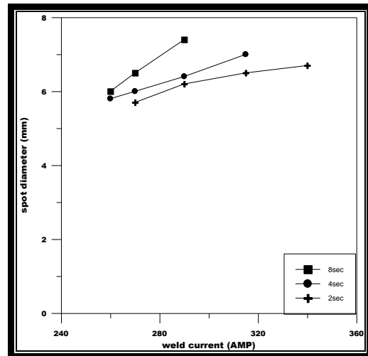
الشكل (٨) تأثير التيار في قطر نقطة اللحام لسمك 4mm مع استخدام غاز CO 2 ولازمان مختلفه
