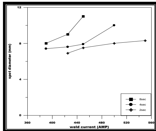
الشكل (٩) تأثير التيار في قطر نقطة اللحام لسمك 6 mm مع استخدام غاز CO 2 ولازمان مختلفه
