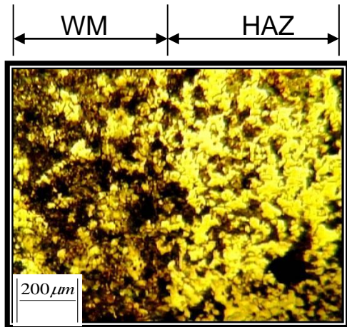
الشكل (٢١) منطقة اللحام (WM) والمنطقة المتأثرة بالحرارة (HAZ) لعينه سمك (2mm) ولزمن (8sec) وغاز CO 2
