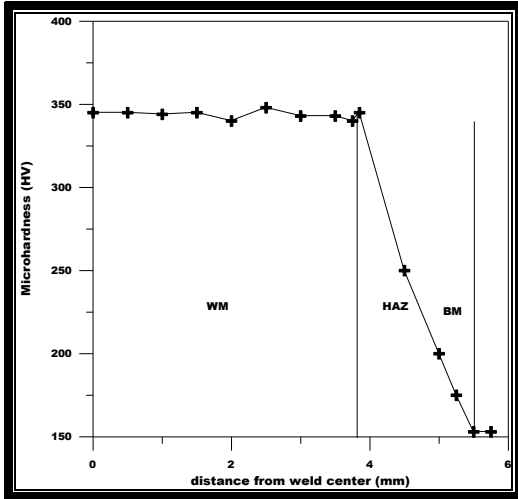
الشكل (15) يمثل منحنى الصلادة الدقيقة لسمك 4mm باستخدام غاز CO 2 وعند زمن ٤ ثانية
