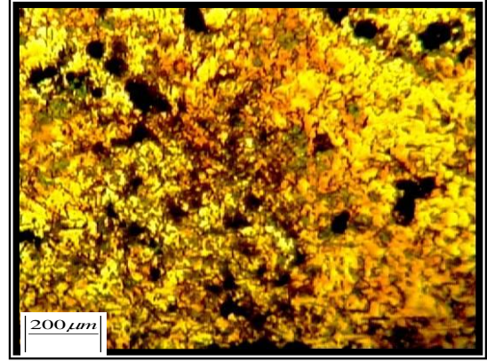
الشكل (٢٥) لمعدن اللحام (WM) ولسمك (6mm) ولزمن (8sec) وباستخدام غاز Ar
