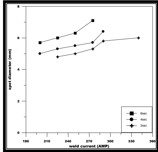
الشكل (١١) تأثير التيار في قطر نقطة اللحام لسمك 4mm مع أستخدام غاز Ar ولازمن مختلفه
