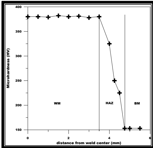
الشكل (16) يمثل منحنى الصلادة الدقيقة لسمك 4mm باستخدام غاز Ar وعند زمن ٤ ثانية
