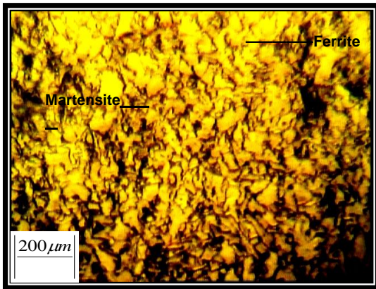
الشكل (٢٤-٤) صورة لمعدن اللحام (WM) ولسمك (4mm) ولزمن (4sec) وبأستخدام غاز (Ar)
