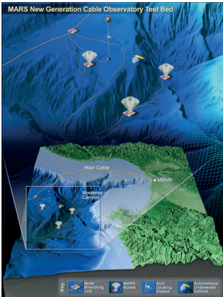
Fig. 9. MARS Observatory.
