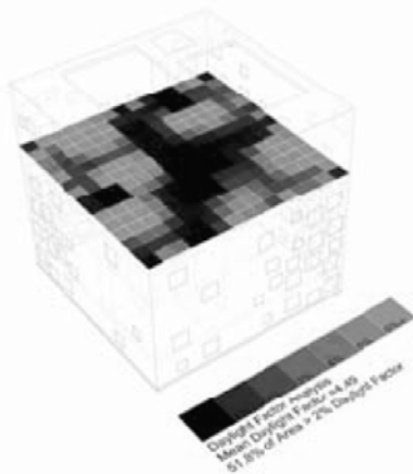
Gambar 5. Hasil varian tunggal: Daylight Factor.
