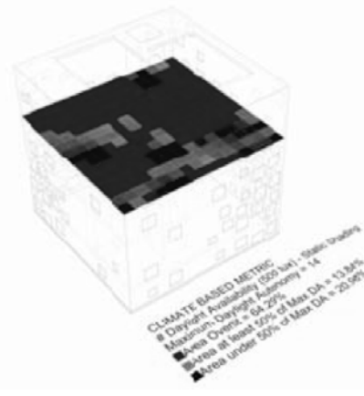
Gambar 6. Hasil varian tunggal: Daylight Availability
