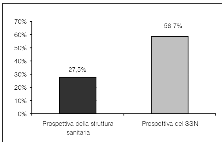
Figura 1 Analisi di sensibilità - Analisi del valore-soglia - Aumento percentuale del costo di fludarabina fosfato p.o. che eguaglia il costo per ciclo terapeutico di 5 giorni con fludarabina fosfato e.v. e fludarabina fosfato p.o.
