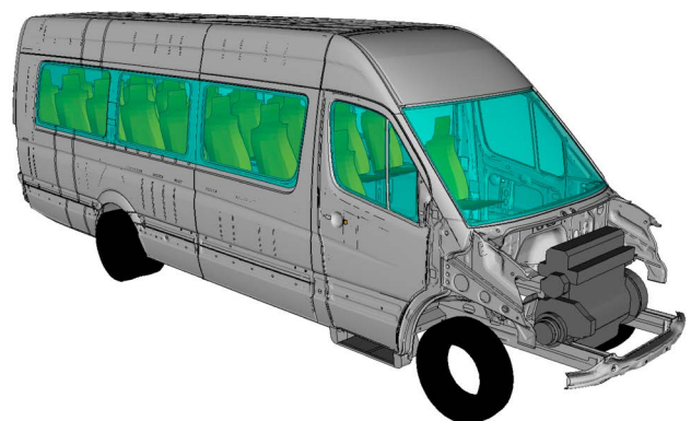
FIGURE 3: Van type of vehicle OBRÁZEK 3: Autobus založený na podvozku dodávky
