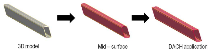
FIGURE 6: Pillar FEM model preparations OBRÁZEK 6: Příprava MKP modelu sloupku
