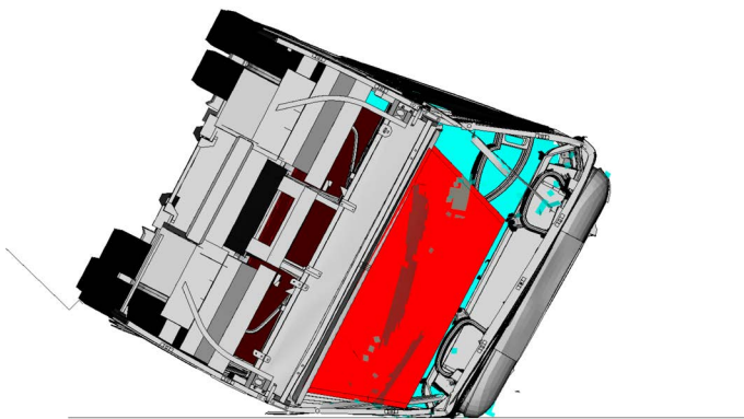
FIGURE 7: Bus rollover OBRÁZEK 7: Převrácení autobusu
