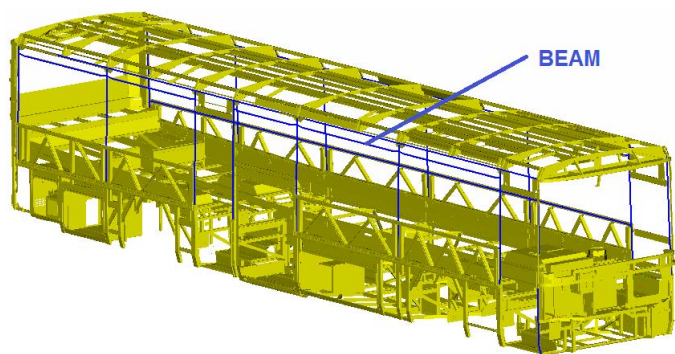
FIGURE 8: T joint with variable pillar height and difference between the PLink joint and connecting of adjacent nodes OBRÁZEK 8: T spoj s proměnnou výškou profilu a rozdíl mezi spojením typu PLink a napojení sousedních uzlů
