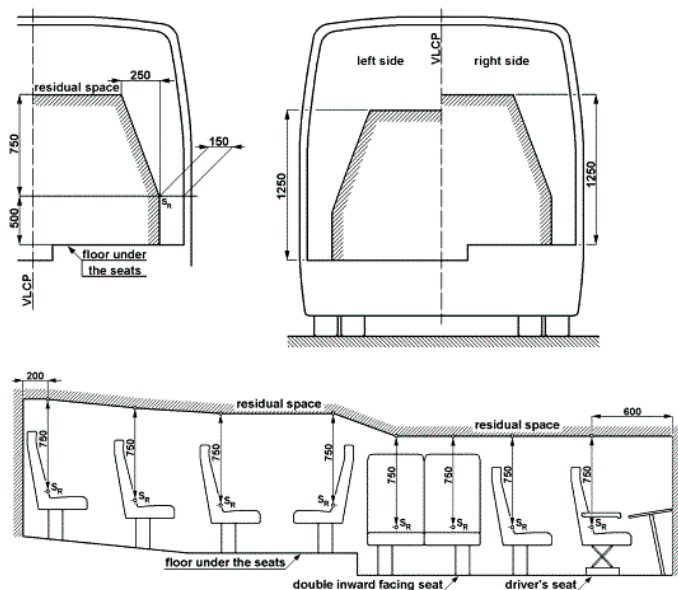
FIGURE 2: Survival space template OBRÁZEK 2: Vymezení prostoru pro přežití
