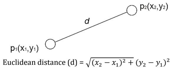
Figure 5. The Euclidean distance (d)
